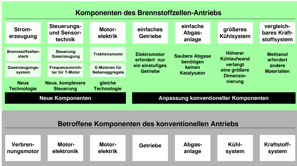
Abbildung 2: Veränderungen durch die Brennstoffzelle gegenüber einem konventionellen Fahrzeug im Überblick (Demuß, 2000)
